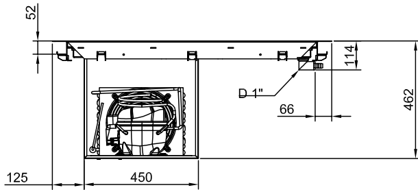
Zij aanzicht
