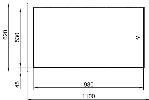
Boven aanzicht
